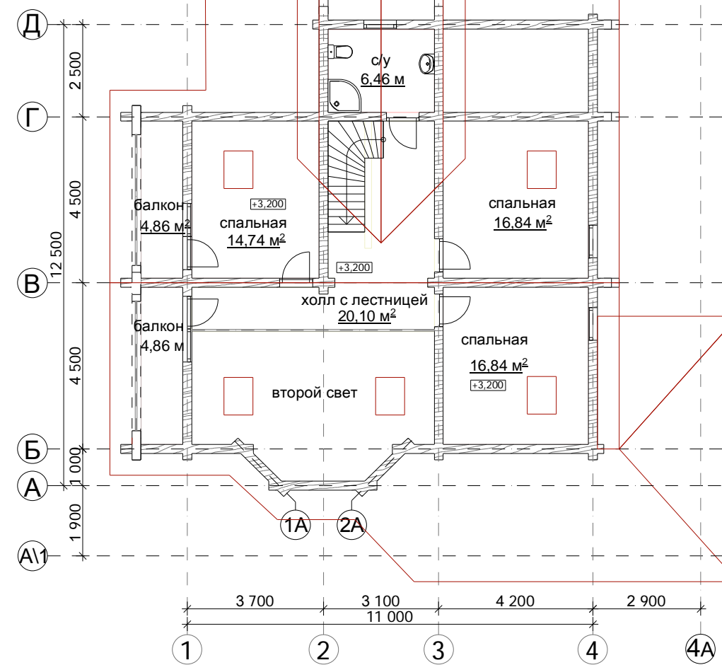
План 2-ого этажа
